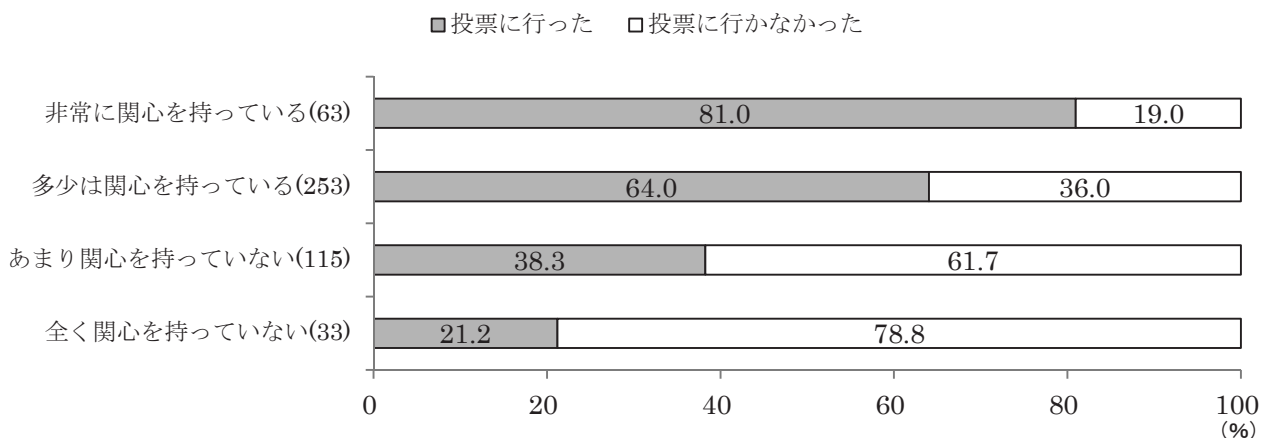
図 4-13 政治関心と投票参加率（20～30 歳代）
