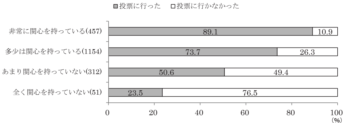
図 4-13 政治関心と投票参加率（20～30 歳代）
