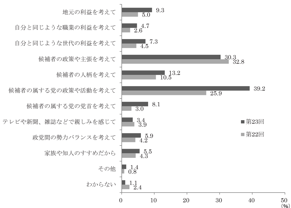
図6-2 選挙区選挙で考慮した点（複数回答）
