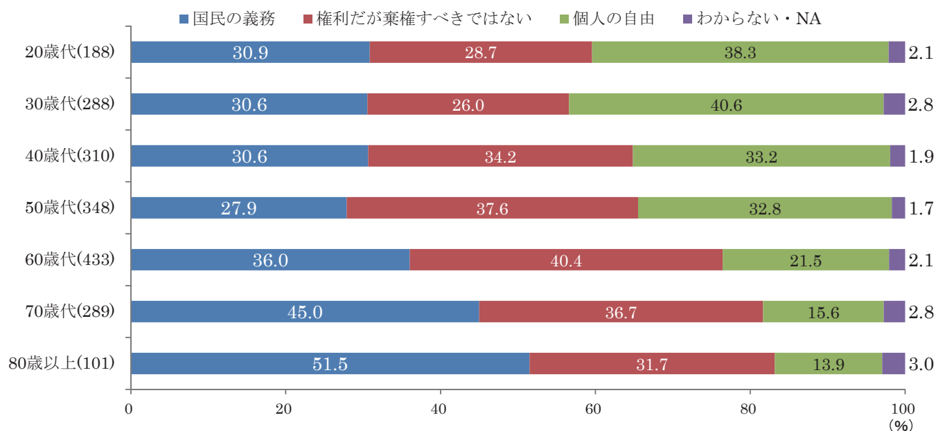
図 3-6 投票に対する意識（年代別）
