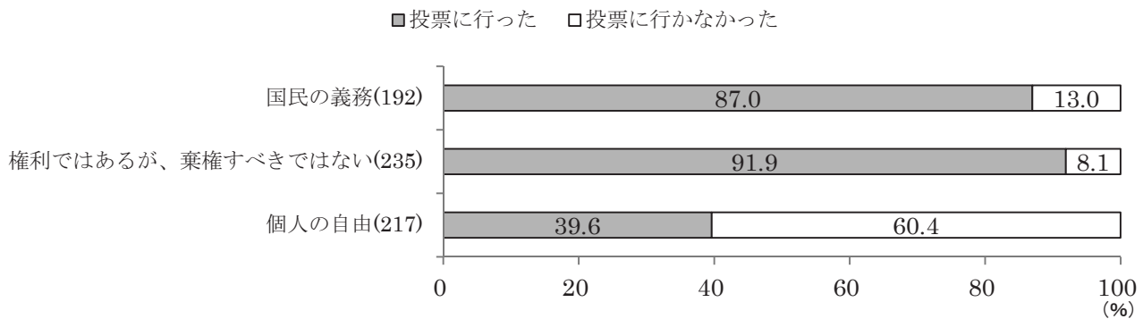
図 4-19 投票に対する考えと投票参加率（60 歳以上）
