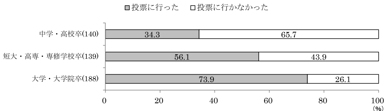
図 4-3 学歴と投票参加率 (20~30 歳代)
