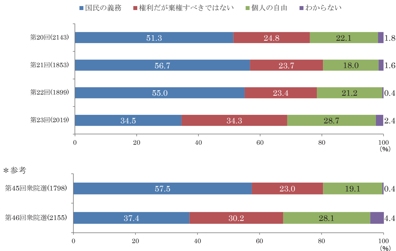
図 3-5 投票に対する意識
