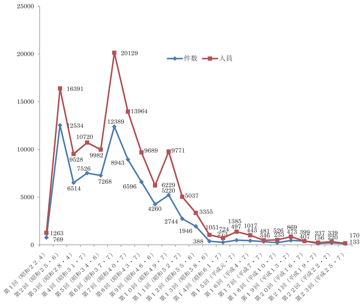
図 2-5 選挙違反検挙数の推移
