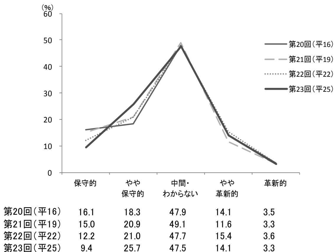
図7-1 イデオロギーの変化
